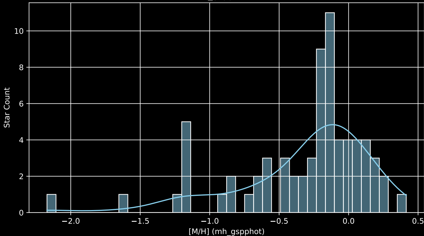
GALAH DR4 Field: [-2] [M/H] (mh_gspphot) (n= 69)
