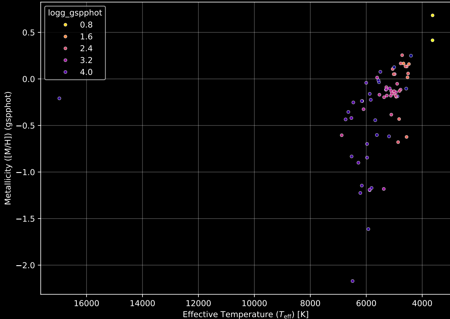
GALAH DR4 Field: [-2] Stellar Population Parameters (n= 70)
