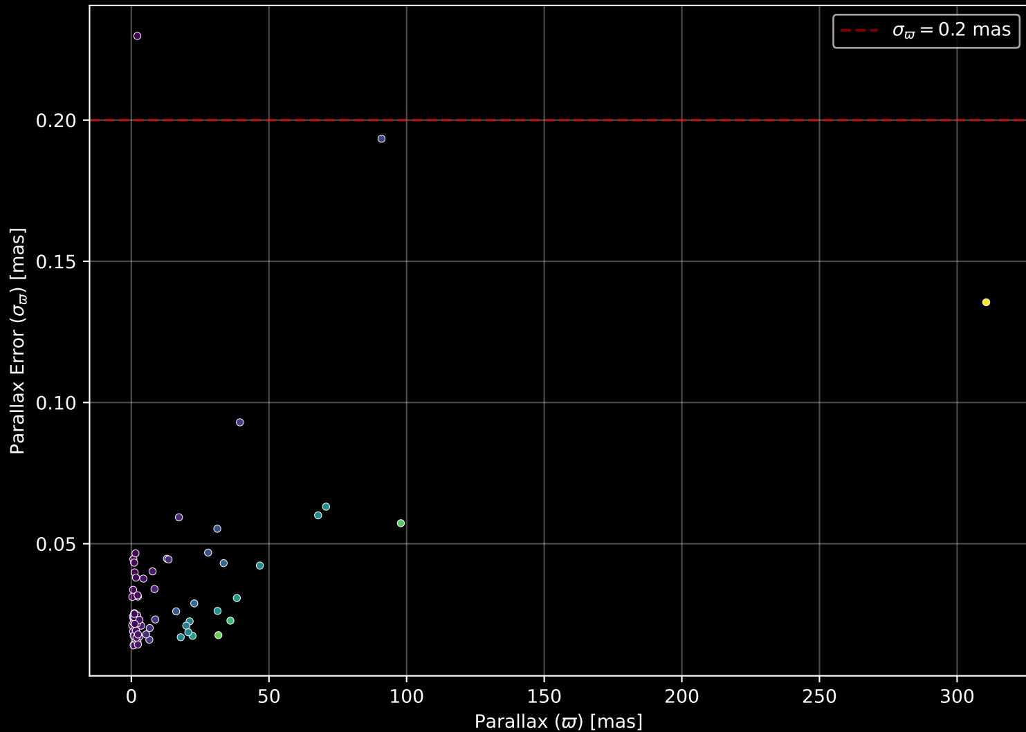
GALAH DR4 Field: [-2] Parallax Quality (n= 70)
